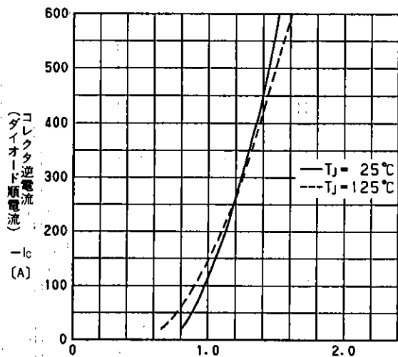
エミッタ・コレクタ間電圧 V_{Eco} (V) (ダイオード順電圧) 高速フリーホイーリングダイオード順電圧特性 Forward Voltage of Free Wheeling Diode
