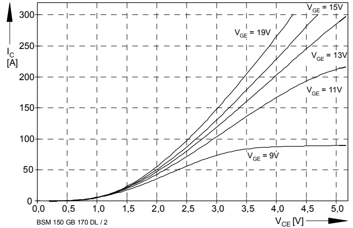
Bild / Fig. 2 Ausgangskennlinienfeld (typisch) / Output characteristic (typical) I_C = f(V_{CE}) T_j = 125^\circ\text{C}
