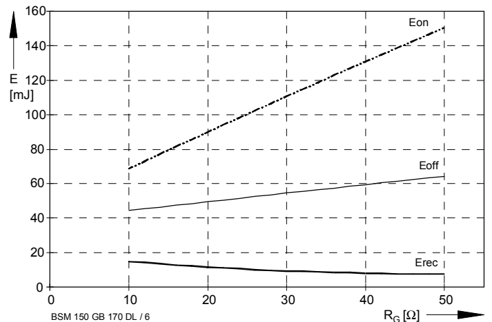
Bild / Fig. 6 Schaltverluste (typisch) / Switching losses (typical) E_{on} = f(R_G) , E_{off} = f(R_G) , E_{rec} = f(R_G) I_C = 150\text{A} , V_{CE} = 900\text{V} , T_j = 125^\circ\text{C}
