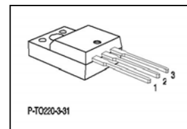
TO220 FP
